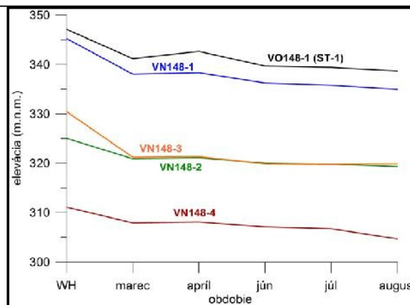
Obr. 3 Časový vývoj HPV v okolí skládky
