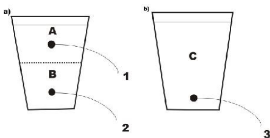
Obr. 1 Schéma lyzimetrických pokusov a) experiment – Zemianske Kostolany, b) experiment – Čereňany; A) vrstva pôdy, B) vrstva elektrárenského popola, C) zmiešaná vrstva nehomogénnej pôdy a elektrárenského popola; 1, 2) a 3) lyzimetrické (rhizónové) vzorkovače
