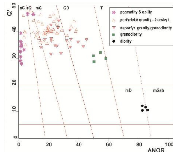
Obr. 3 Diagram Q'-\text{ANOR} s využitím mezonormy na detailnejšie odlíšenie jednotlivých typov granitoidov.
