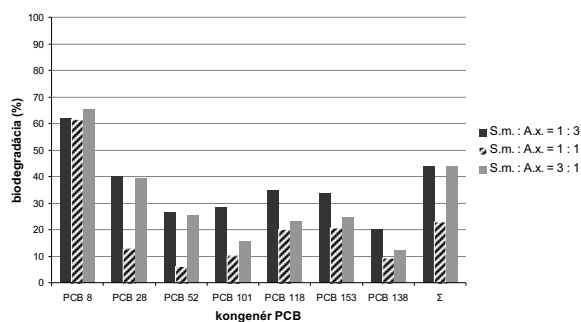
Obr. 3 Biodegradácia kongenérův PCB konzorciom S.maltophilia + A.xylosoxidans .
