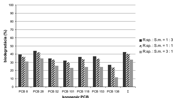
Obr. 2 Biodegradácia kongenérův PCB konzorciom S.maltophilia + A.xylosoxidans .
