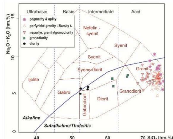
Obr. 2 TAS klasifikačný diagram granitoidov Žiaru.
