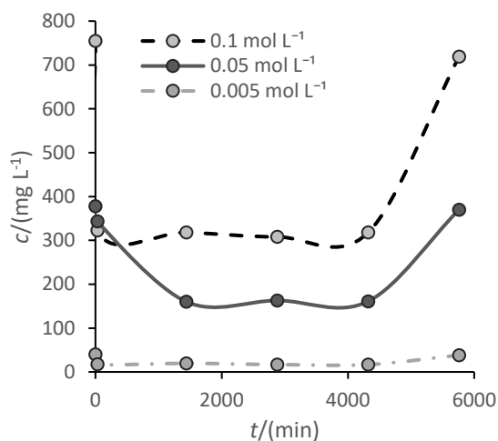
Obr. 1 Zmeny koncentrácie selénu v roztoku počas kryštalizácie goetitu
