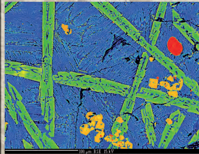
Kryštály wollastonitu v troskovom metalurgickom odpade, BSE snímka (EZ Kovohuty Kropachy, foto. R. Demko)
