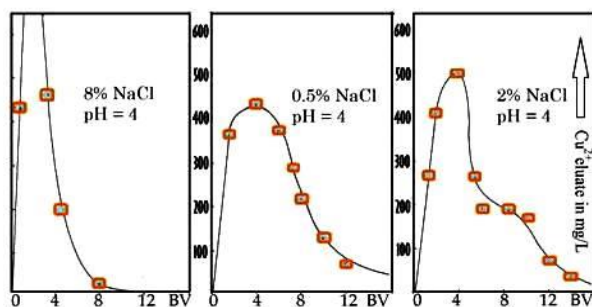
Obr. 2a Desorpce Cu – iónov z modelových kolón roztokmi NaCl
