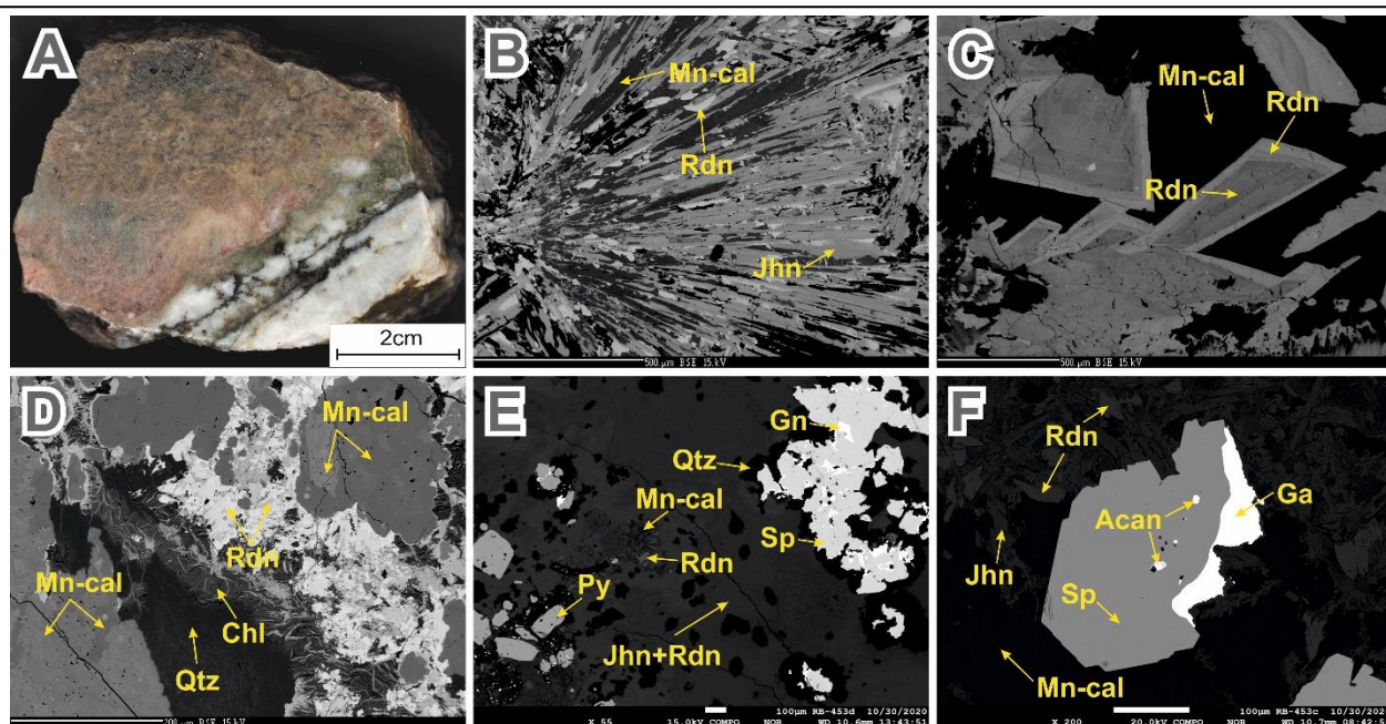
Obr. 1 Fotodokumentácia a BSE snímky študovanej Mn-mineralizácie: A) Vzorka s charakteristickými agregátmi johannsenitu a bieleho karbonátu s tmavými žilkami klinozoisitu. B) Radiálne lúčovitý johannsenit (sivý), intímne prerastený s rodonitom (biely) a Mn-kalcitom (tmavosivý). C) Zonálny rodonit v Mn-kalcite má oscilačnú a sektorovú zonálnosť, spôsobenou zmenou obsahu Ca a Mn. D) Vlákňitý chlorit v asociácii s rodonitom, kremeňom a Mn-kalcitom. E) Resorbované zrná kremeňa asociujúce so sulfidmi v jemnozrnej zmesi Mn-minerálov. F) Inklúzie akantitu vo sfalerite v asociácii s galenitom v zmesi Mn-minerálov.
