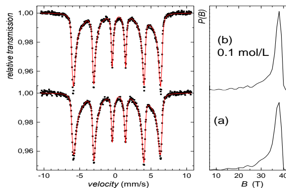
Obr. 2 Mössbauerove spektrá syntetizovaných vzoriek goethitu bez selénu (a) a s najvyššou koncentráciou selénu (b)
