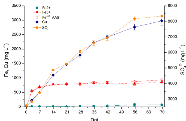
Obr. 1 Bakteriálne lúhovanie tetraedritového koncentrátu s obsahom sideritu. Grafy zobrazujú priemerné hodnoty z 2 paralelných experimentov ± SD ( At. ferrooxidans )
