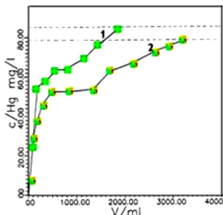
Obr. 2b Profilové krivky mordenitovým lôžkom pri prítoku 9,6 V/vo roztoku \text{HgCl}_2 (1), \text{Hg}(\text{CH}_3\text{COO})_2 (2)
