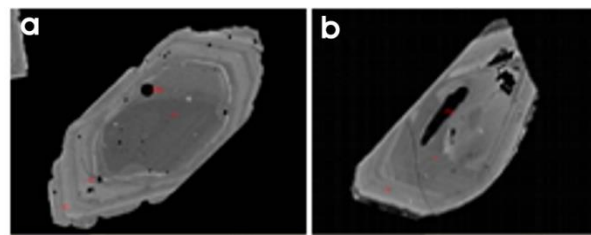
Obr. 4 a) Oscilačne zonálny magmatický zirkón (Zabiedovo); b) neskoromagmatický zirkón (Krivá) uzatvára pyrit.
