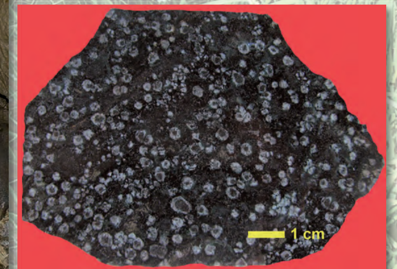
Oceánsky bazalt typu E-MORB klátovskej skupiny metamorfovaný pôvodne na eklogit, neskôr retrográdne premenený na granatický amfibolit. Predstavuje relikt po cenerijskej sutúre ordovického veku. Lokalita: Dobšiná, Malá Vičia dolina (foto. P. Ivan)
