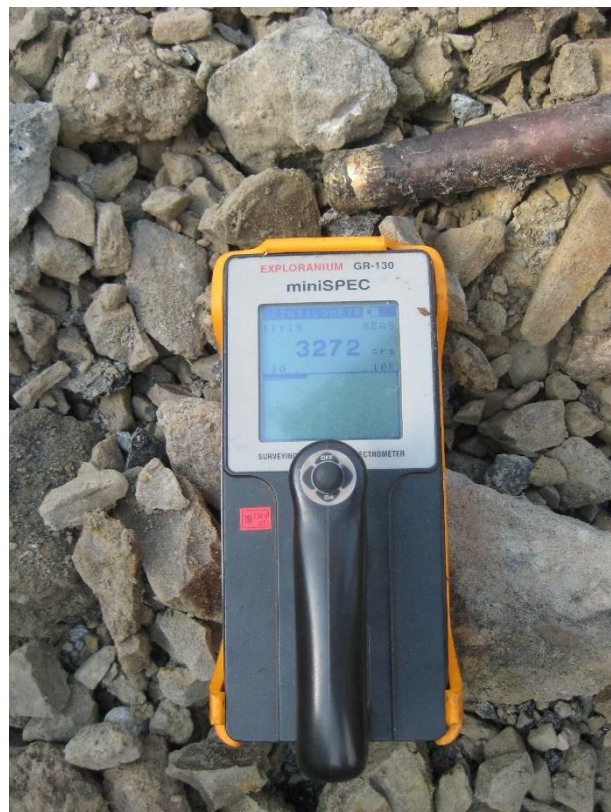
Obr. 4 Mosazná trubka se zářičem – 3\,272 \mu\text{Gy}\cdot\text{h}^{-1}
