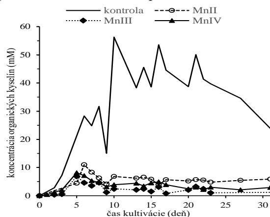
Obr. 3 Zmeny koncentrácie produkovaného oxalátu v živnom médiu počas statickej kultivácie mikroskopической vláknitej huby A. niger
