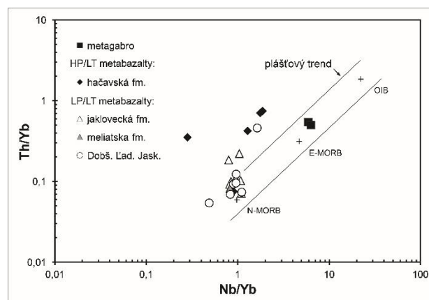
Obr. 3 Metagabrá z hačavskej formácie v diagrame \text{Nb}/\text{Yb} vs. \text{Th}/\text{Yb} v porovnaní s metabazaltami rôznych meliatských formácií. Ich geochemická blízkosť typu E-MORB ich odlišuje od ostatných metabazitov meliatika, ktoré sú blízke oceánskeho typu N-MORB alebo horninám ostrovných oblúkov
