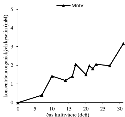
Obr. 5 Zmeny koncentrácie produkovaného octanu v živnom médiu počas statickej kultivácie mikroskopkej vláknitej huby A. niger
