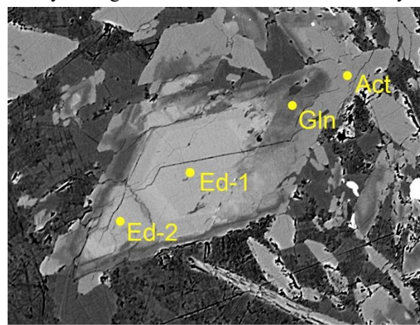
Obr. 1 Koncentricky zonálny amfibol v metagabre v spätne odrazených elektrónoch so zónami edenitu (Ed), glaukofánu (Gln) a aktinilitu (act)
