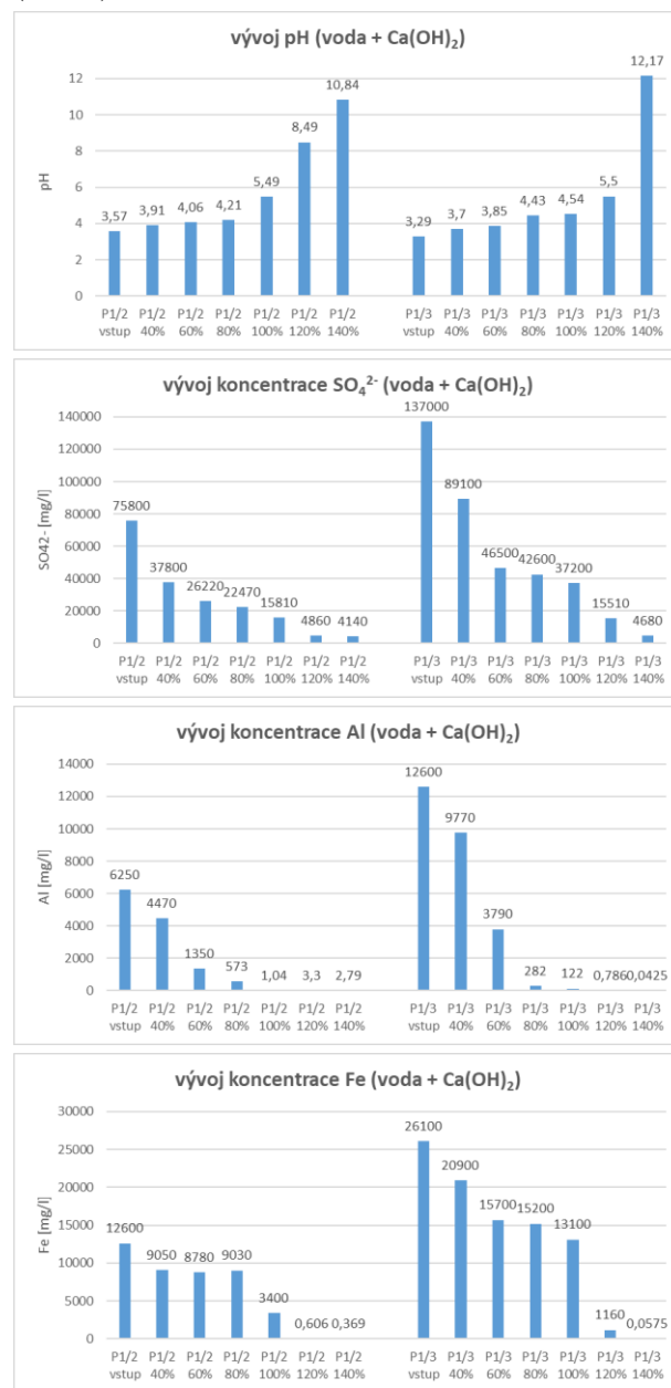
Obr. 3 Výsledky laboratorních experimentů neutralizace kontaminované podzemní vody hydroxidem vápenatým.
