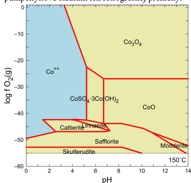
Obr. 3 Fázový diagram systému Co-As-S-O-H pri 150 °C a \log a(\text{As}_{\text{tot}}) = -2 , \log a(\text{Co}_{\text{tot}}) = -3 , \log a(\text{S}_{\text{tot}}) = -3 . Minerály: skutterudit – CoAs 3 , safflorit – CoAs 2 , modderit – CoAs, catterit – CoS 2 , linnaeit – Co 3 S 4 .
