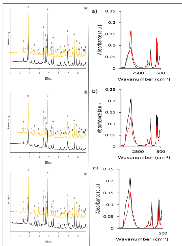
Obr. 1 Výsledky HEXRD analýzy železitých precipitátov vykryštalizovaných v alkalickej roztoku (a) bez Se, (b) upravenej Se(IV) a (c) Se(VI) druhý (čierna čiara) a piaty (žltá čiara) deň dozrievania (Symboly „o“ označujú charakteristické XRD obrazce pre goethit ( \alpha\text{-FeOOH} ) a symboly „•“ označujú vyzrážaný dusičnan draselný ( \text{KNO}_3 )) (vľavo). ATR-FTIR spektrá železitých precipitátov v alkalickej roztokoch (a) bez Se, (b) upravenej Se(IV) a (c) Se(VI) druhý (čierna čiara) a piaty (červená čiara) deň dozrievania (vpravo).
