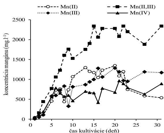
Obr. 1 Zmeny koncentrácie celkového rozpusteného mangánu v živnom médiu počas statickej kultivácie mikroskopической vláknitej huby A. niger v prítomnosti rôznych oxidov mangánu
