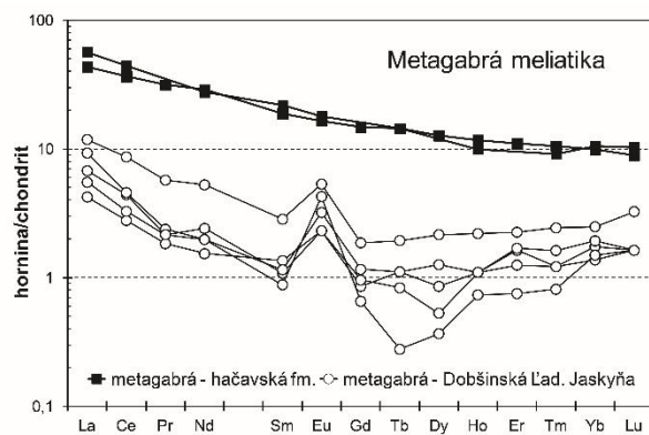
Obr. 2 Chondritovo normalizované obrazy prvkov skupiny vzácnych zemín v metagabrách z hačavskej formácie porovnané s obrazmi valúnov metagabier meliatika z kriedových konglomerátov z Dobšinskej Ľadovej Jaskyne.
