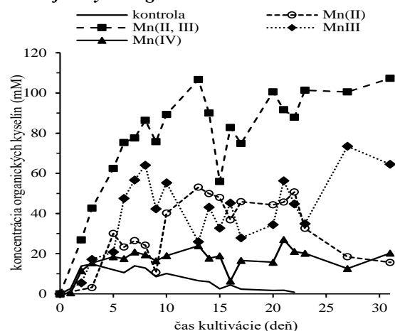
Obr. 4 Zmeny koncentrácie produkovaného glukonátu v živnom médiu počas statickej kultivácie mikroskopической vláknitej huby A. niger
